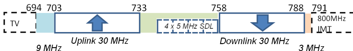
Obr. 2 – Předpokládané uspořádání pásma 700 MHz pro komerční IMT, kompatibilní s využitím v regionech Asie, Austrálie a Jižní Ameriky
