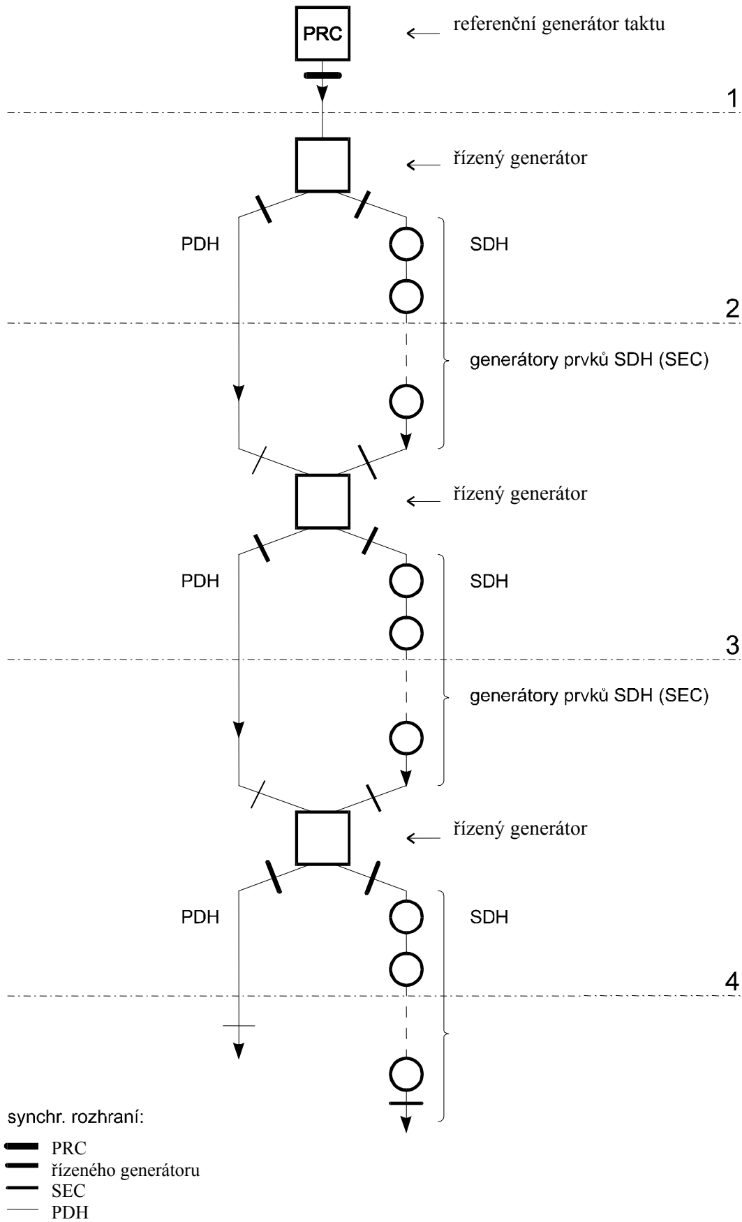
Obr. 3 - Využití multiplexů PDH, SDH. Synchronizační rozhraní
