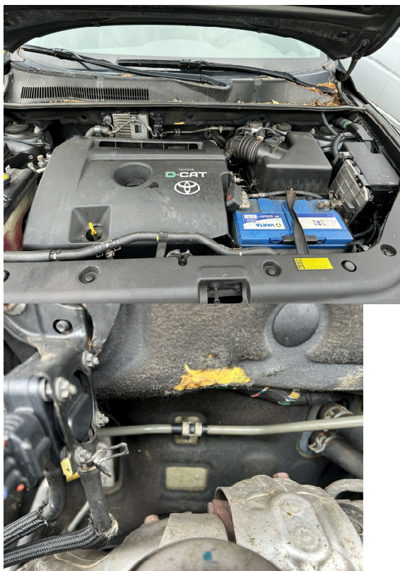
Protihluková výpň poškozena od hlodavců, možnost poškození elektroinstalace
