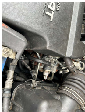
Koroze tělesa vstřikovacího čerpadla, oxidace Al dílů motoru
