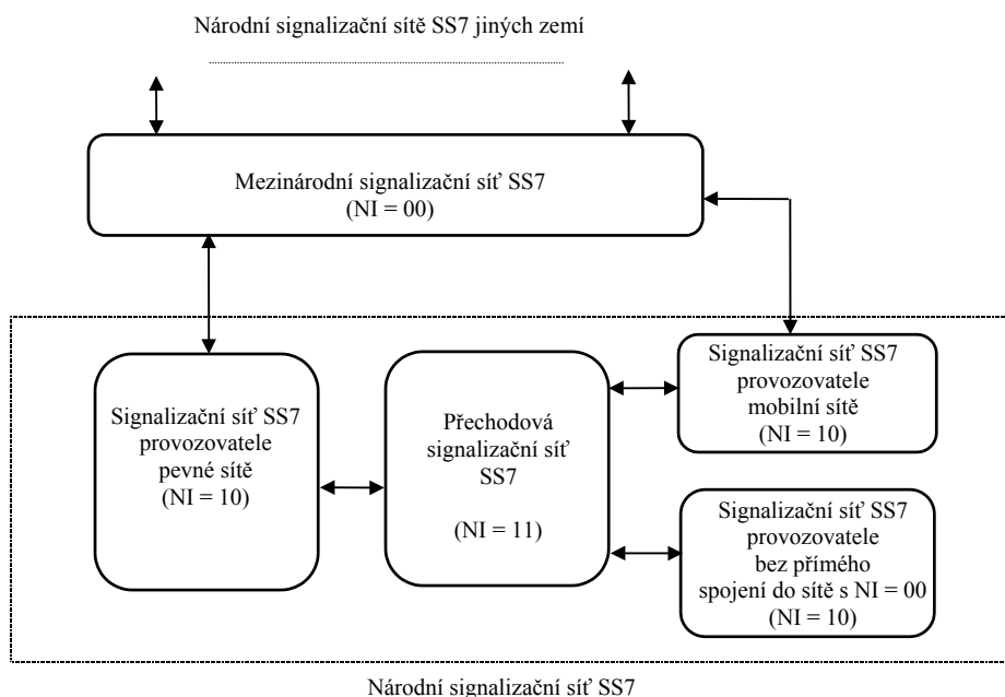
Obr. 1: Obecné uspořádání signalizační sítě SS7“.
