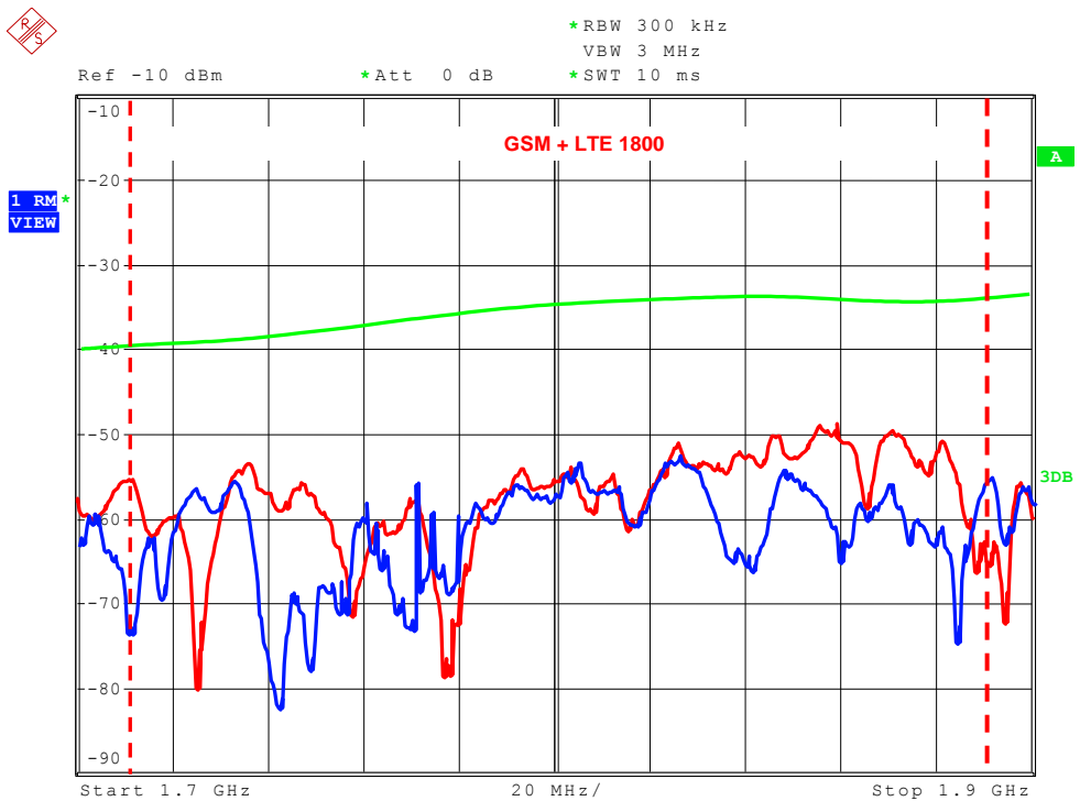
Naměřené hodnoty úrovní signálů v pásmu 1,7-1,9 GHz
