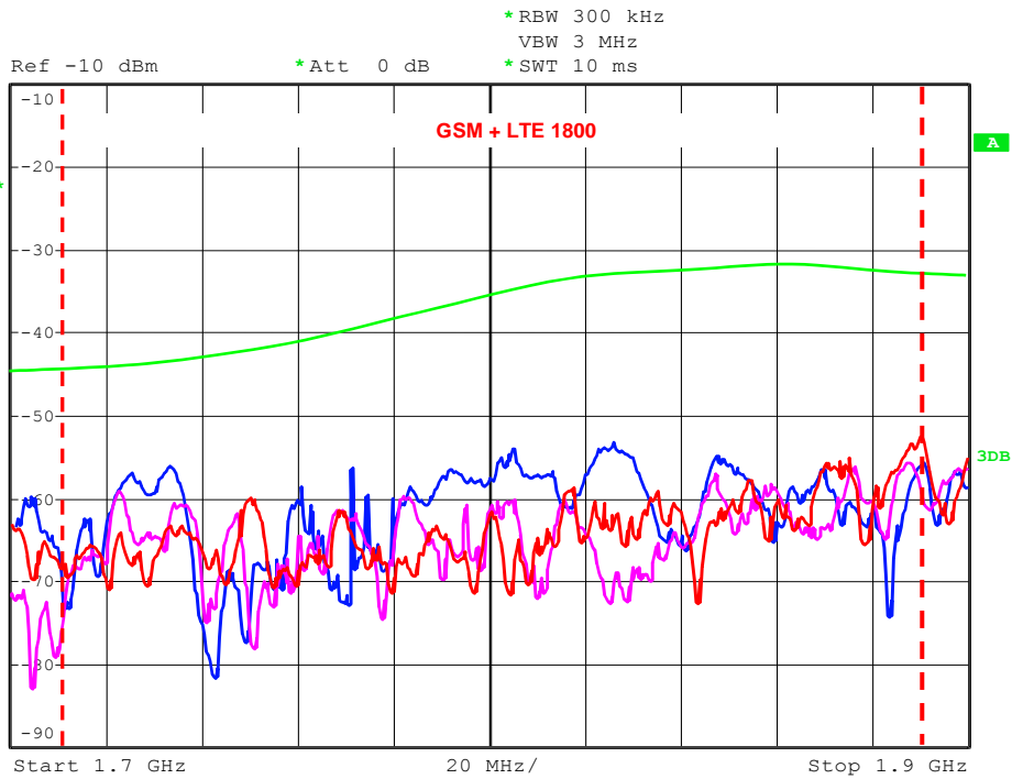
Naměřené hodnoty úrovní signálů v pásmu 1,7-1,9 GHz
