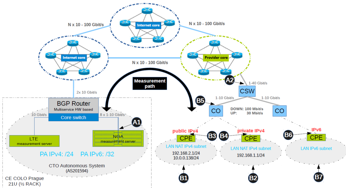
Obrázek P3.2: Měřicí scénáře – NGA síť - příklady
