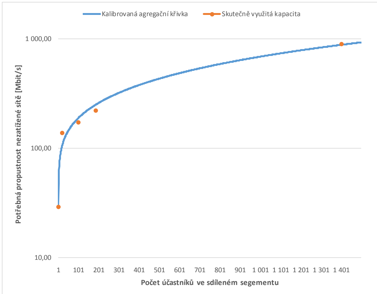
Graf. P2.3: Graf kalibrované agregační křivky s vnesenými body skutečně využití kapacity
